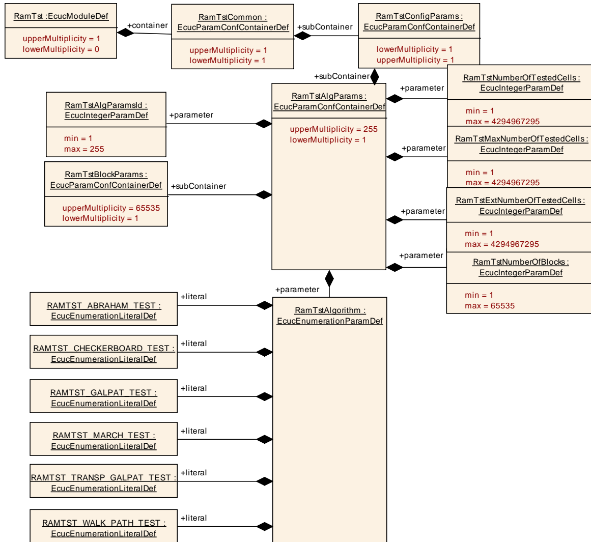
Figure 19: RamTstAlgParams
