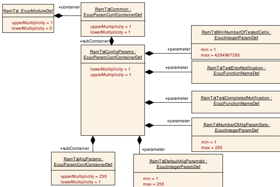
Figure 18: RamTstConfigParams
