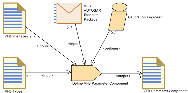
Figure 3.28: Task Define VFB Parameter Component
